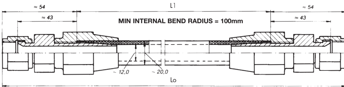
HOSE : Model NP 121 - 8 x L1
